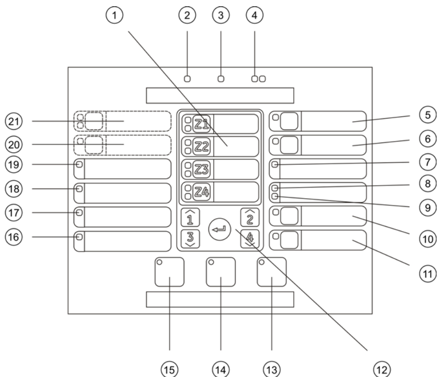
Afbeelding 1: Gebruikersinterface voor twee- en vier-zone bedieningspanelen
